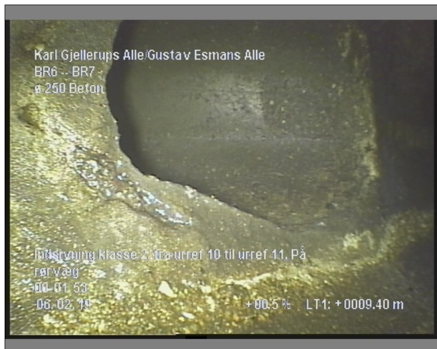
Foto: 7_7A, Medie #: LY19.9007, 00:01:53 9,4m, Indsivning klasse 2, fra urref 10 til urref 11, På rør væg
