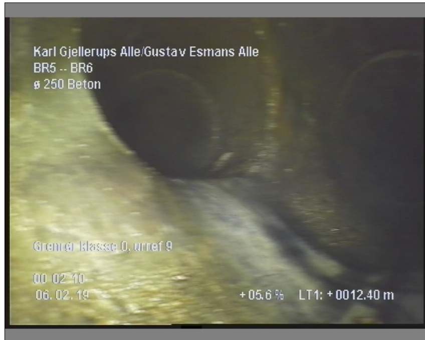
Foto: 6_7A, Medie #: LY19.9007, 00:02:10 12,4m, Grenrør klasse 0, urref 9
