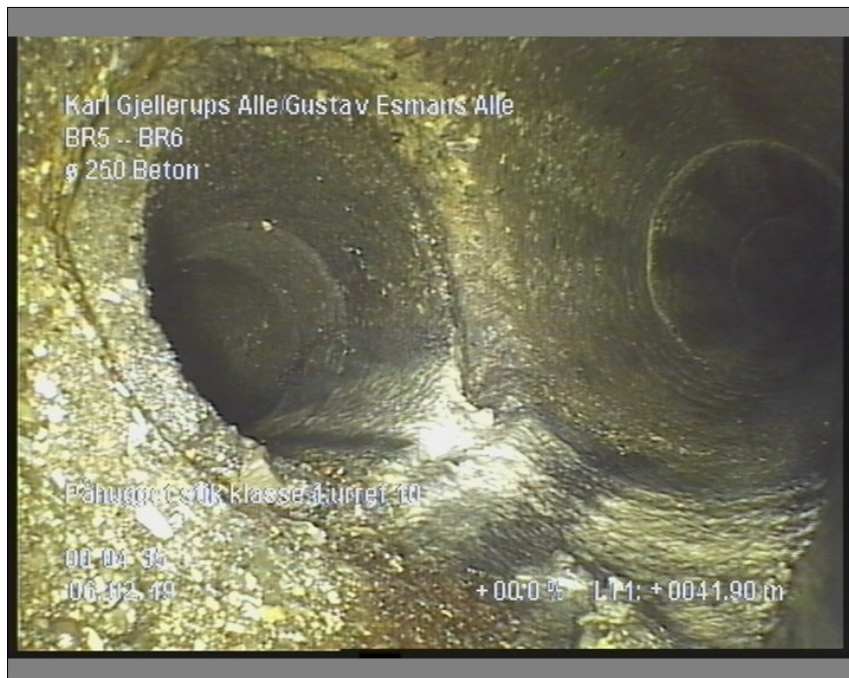
Foto: 6_11A, Medie #: LY19.9007, 00:04:35 41,9m, Påhugget stik klasse 1, urref 10
