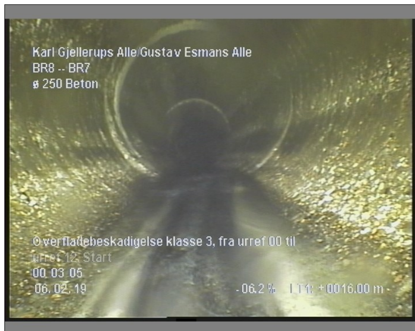
Foto: 8_13A, Medie #: LY19.9007, 00:03:05 16m, Overfladebeskadigelse klasse 3, fra urref 00 til urref 12, Start
