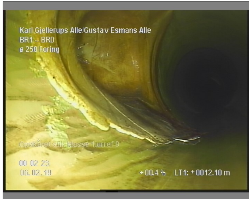
Foto: 3_9A, Medie #:: LY19.9007, 00:02:23 12,1m, Opskåret stik klasse 1,urref 9
