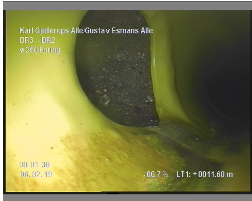
Foto: 4_4A, Medie #: LY19.9007, 00:01:30 11,6m, Opskåret stik klasse 1,urref 9
