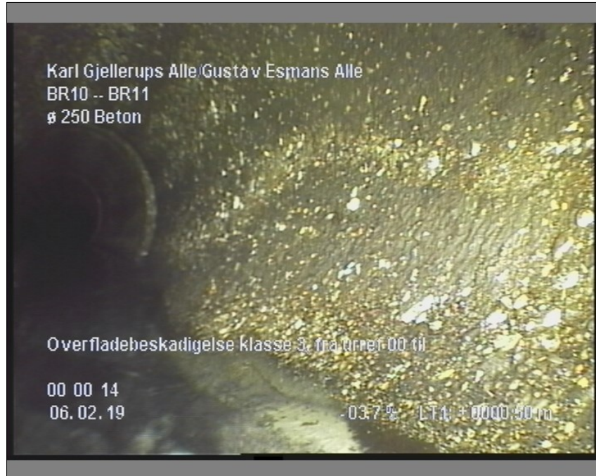
Foto: 10_2A, Medie #: LY19.9007, 00:00:15 0,5m, Overfladebeskadigelse klasse 3, fra urref 00 til urref 12, Start
