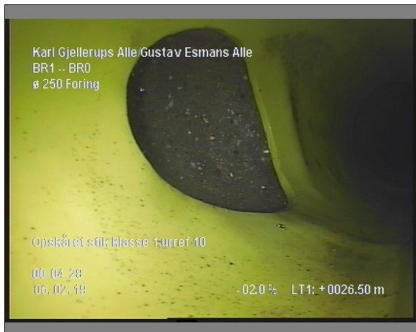
Foto: 3_15A, Medie #:: LY19.9007, 00:04:28 26,5m, Opskåret stik klasse 1,urref 10
