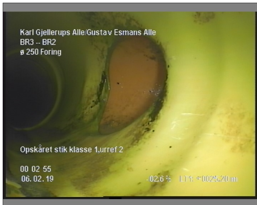
Foto: 4_6A, Medie #: LY19.9007, 00:02:55 25,2m, Opskåret stik klasse 1,urref 2
