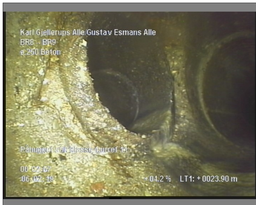
Foto: 11_9A, Medie #:: LY19.9007, 00:02:57 23,9m, Påhugget stik klasse 1,urref 11
